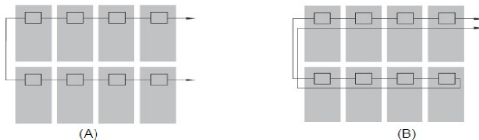
Figura 1: Método de instalação dos cabos CC. (a) Método não permitido para a instalação fotovoltaica (b) Método a ser considerado na instalação fotovoltaica, para minimizar indução de descargas atmosféricas.
