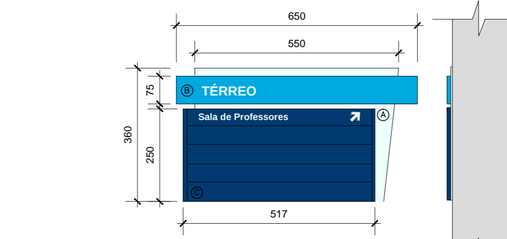
04 SINALIZAÇÃO- PAINEL DIRECIONAL PD.01 ESCALA 1/10
