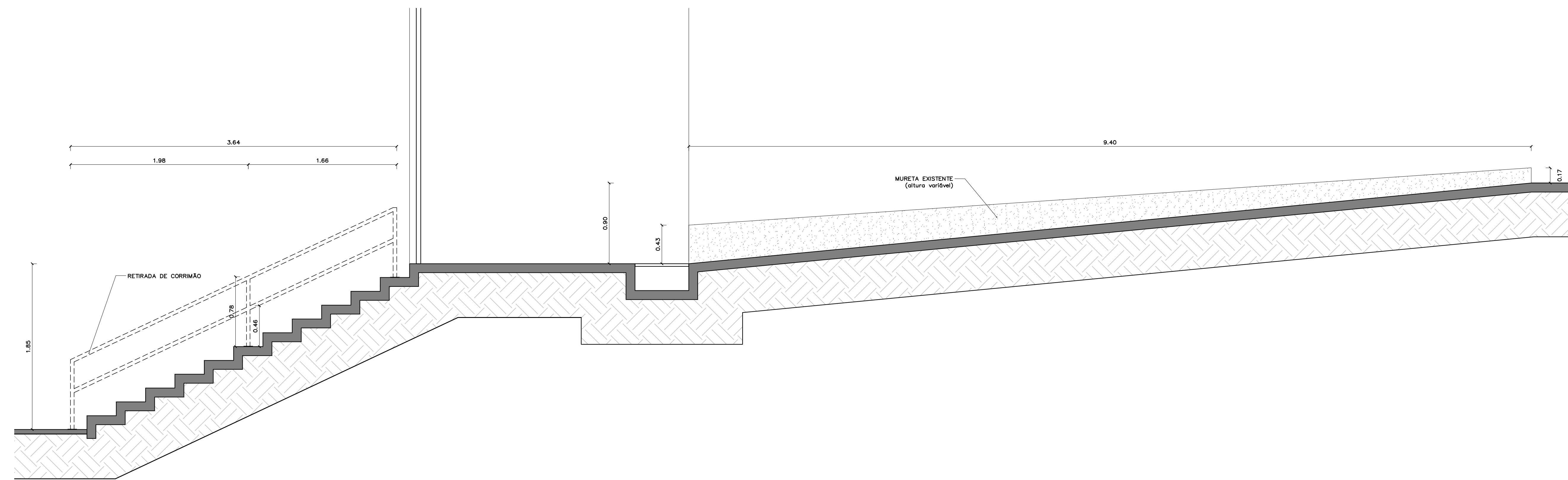
CORTE HH ESCADA 05 E RAMPA 02 ESC: 1:25
