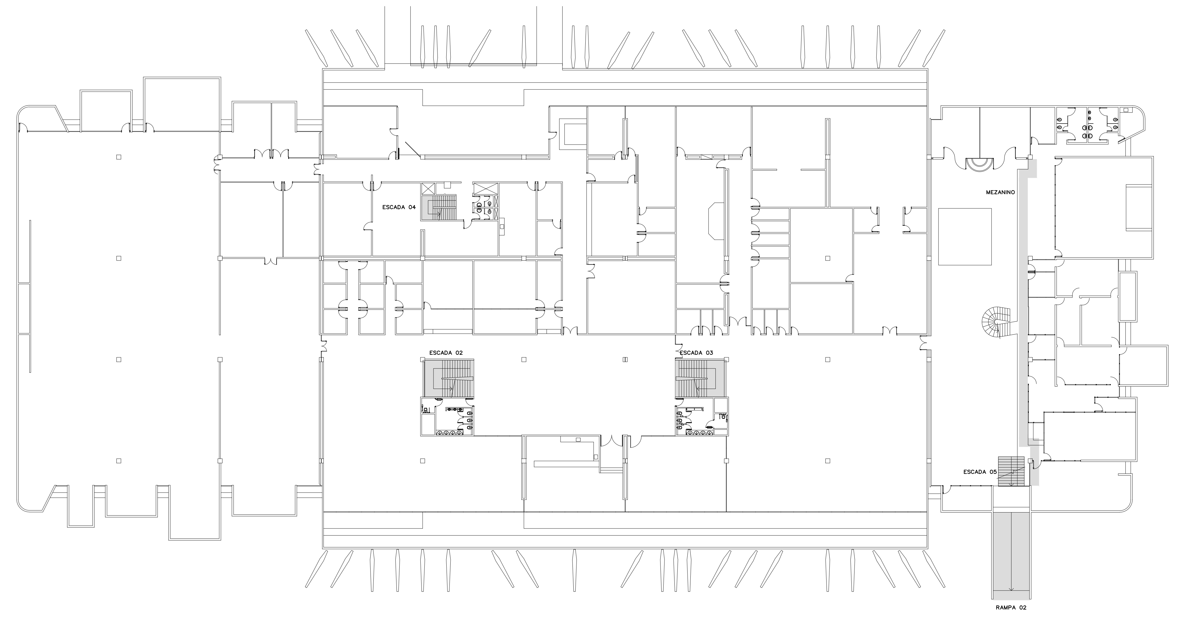
PLANTA DE LOCAÇÃO 1º SUBSOLO ESC.: 1:250
