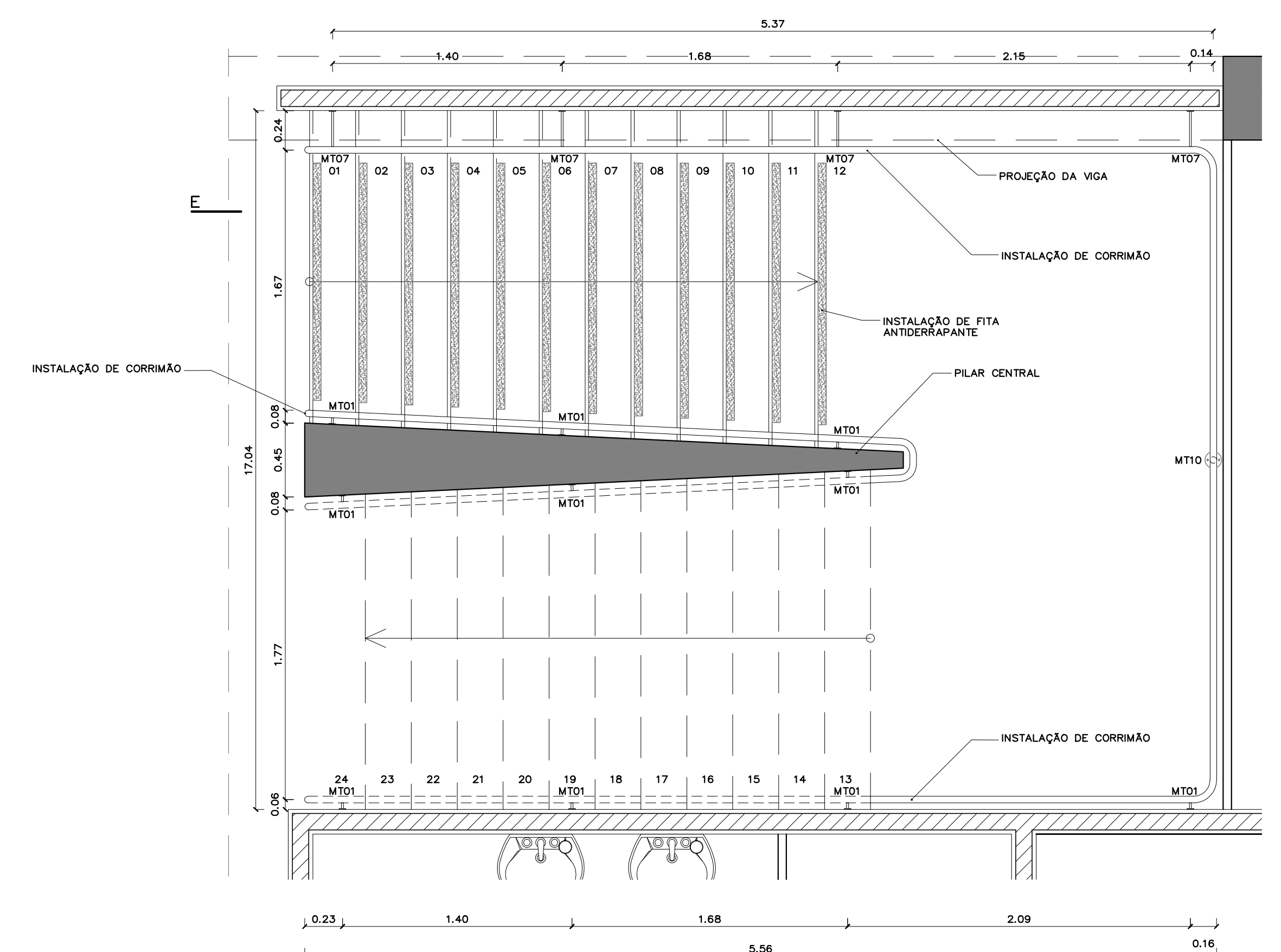
PLANTA BAIXA ESCADAS 02 E 03 (1º SUBSOLO) ESC.: 1:25
