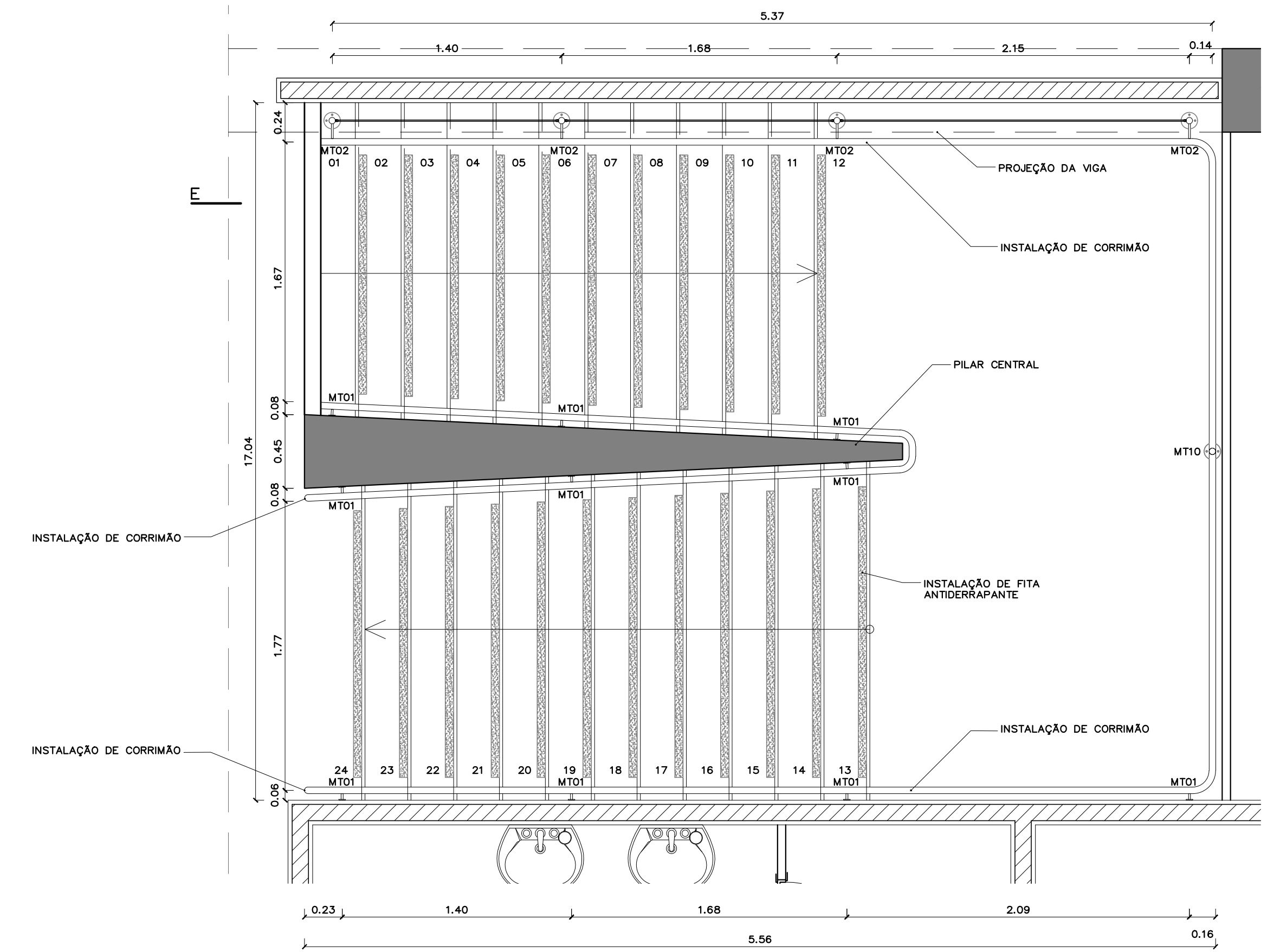
PLANTA BAIXA ESCADAS 02 E 03 (1º PAVIMENTO) ESC.: 1:25
