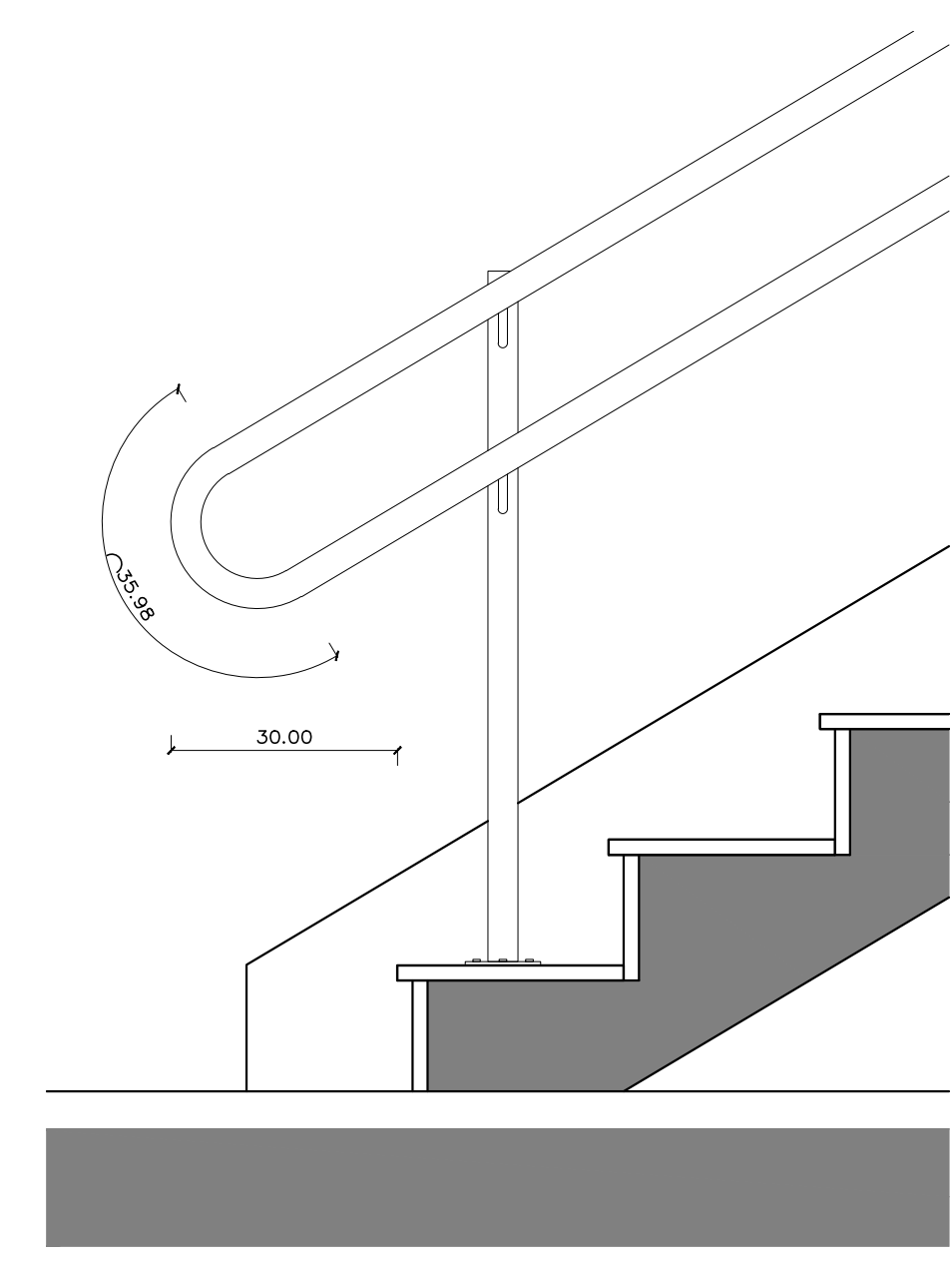
DETALHE CORRIMÃO ESC.: 1:10 OBS.: A FINALIZAÇÃO DE TODOS OS CORRIMÕES SERÁ EM CURVA UNIDAS ÀS QUATRO BARRAS, ULTRAPASSANDO 30cm O ESPELHO DO ÚLTIMO DEGRAU.
