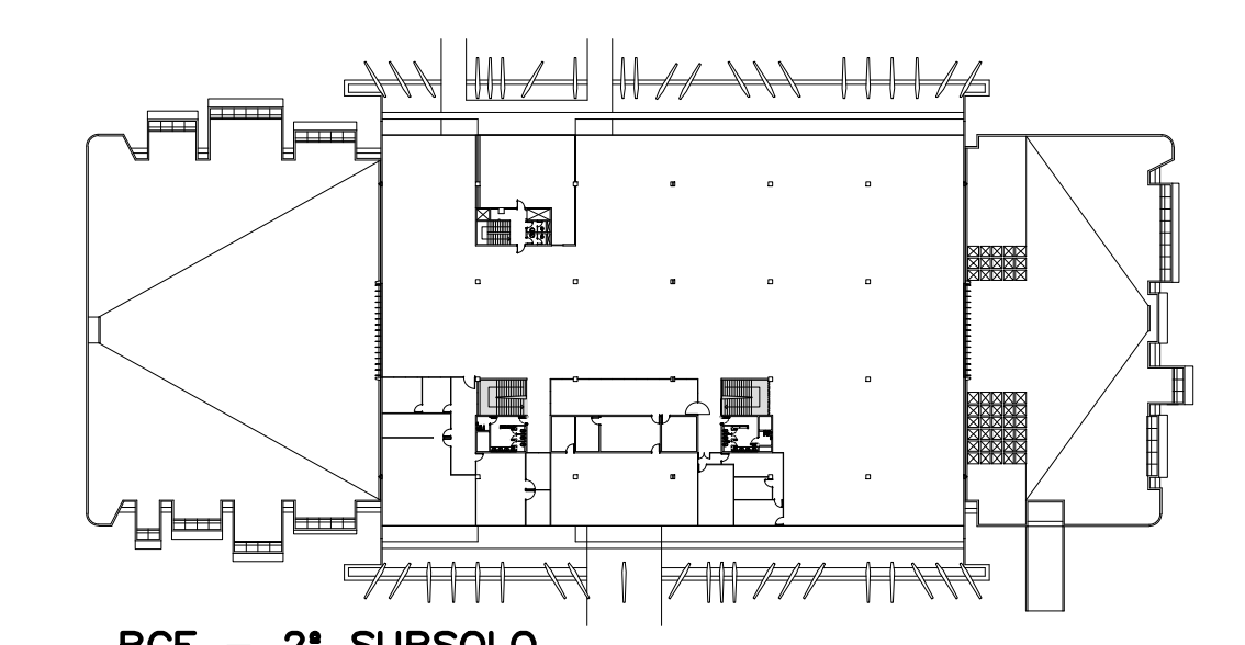
BCE - 2º SUBSOLO ESC.: 1:1000
