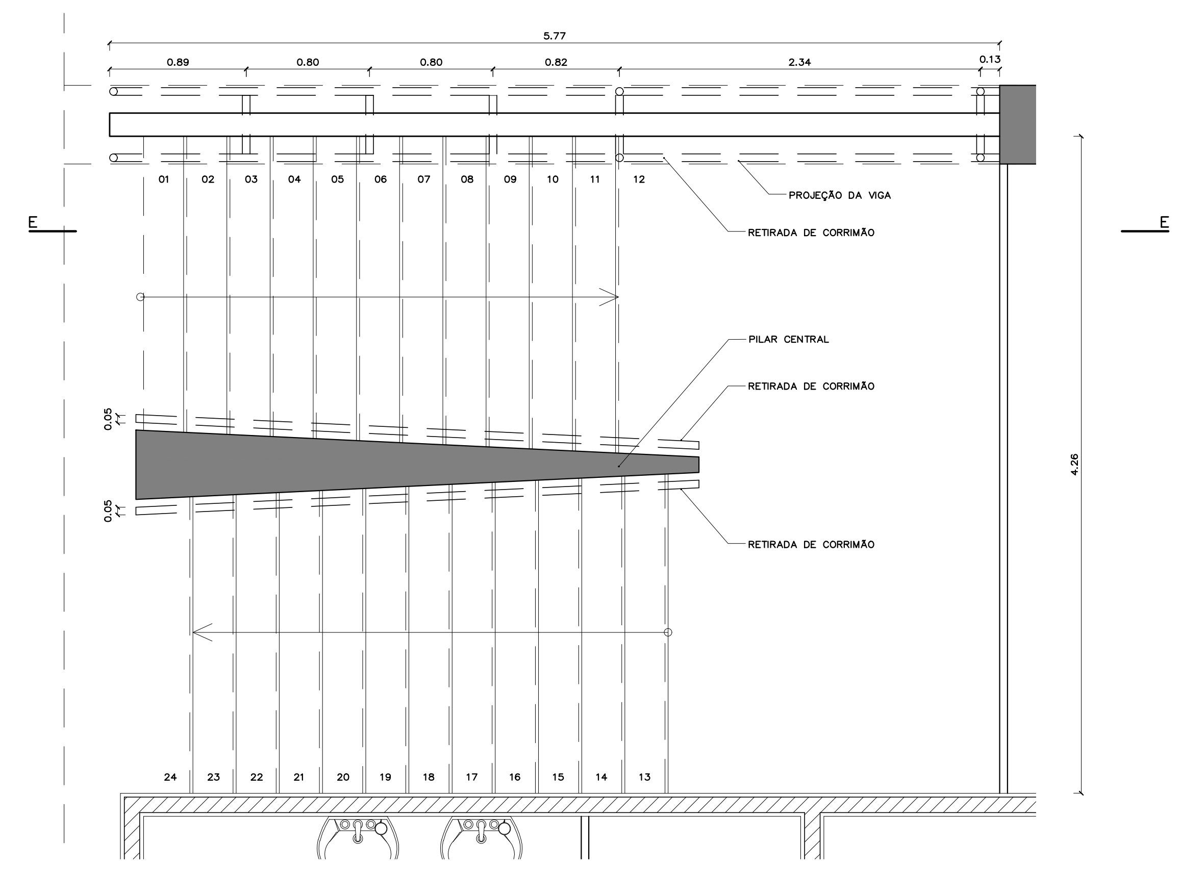
PLANTA DEMOLIR / CONSTRUIR ESCADAS 02 E 03 (TÉRREO) ESC.: 1:25
