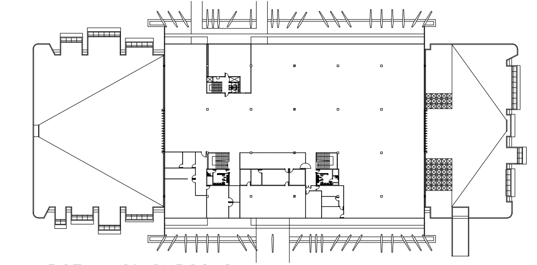
BCE - 2º SUBSOLO ESC: 1:1000
