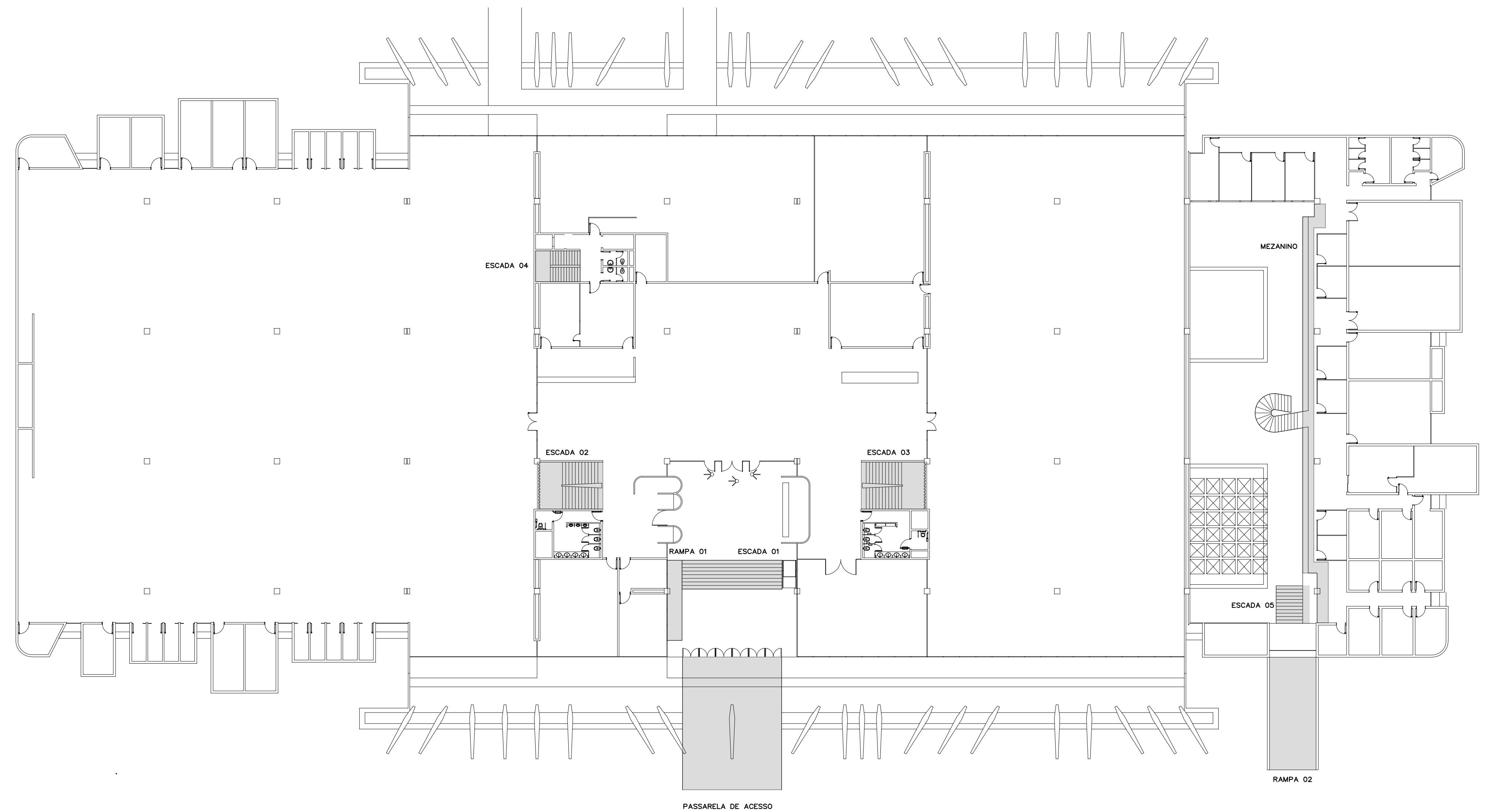
PLANTA DE LOCAÇÃO TERRENO ESC.: 1:250
