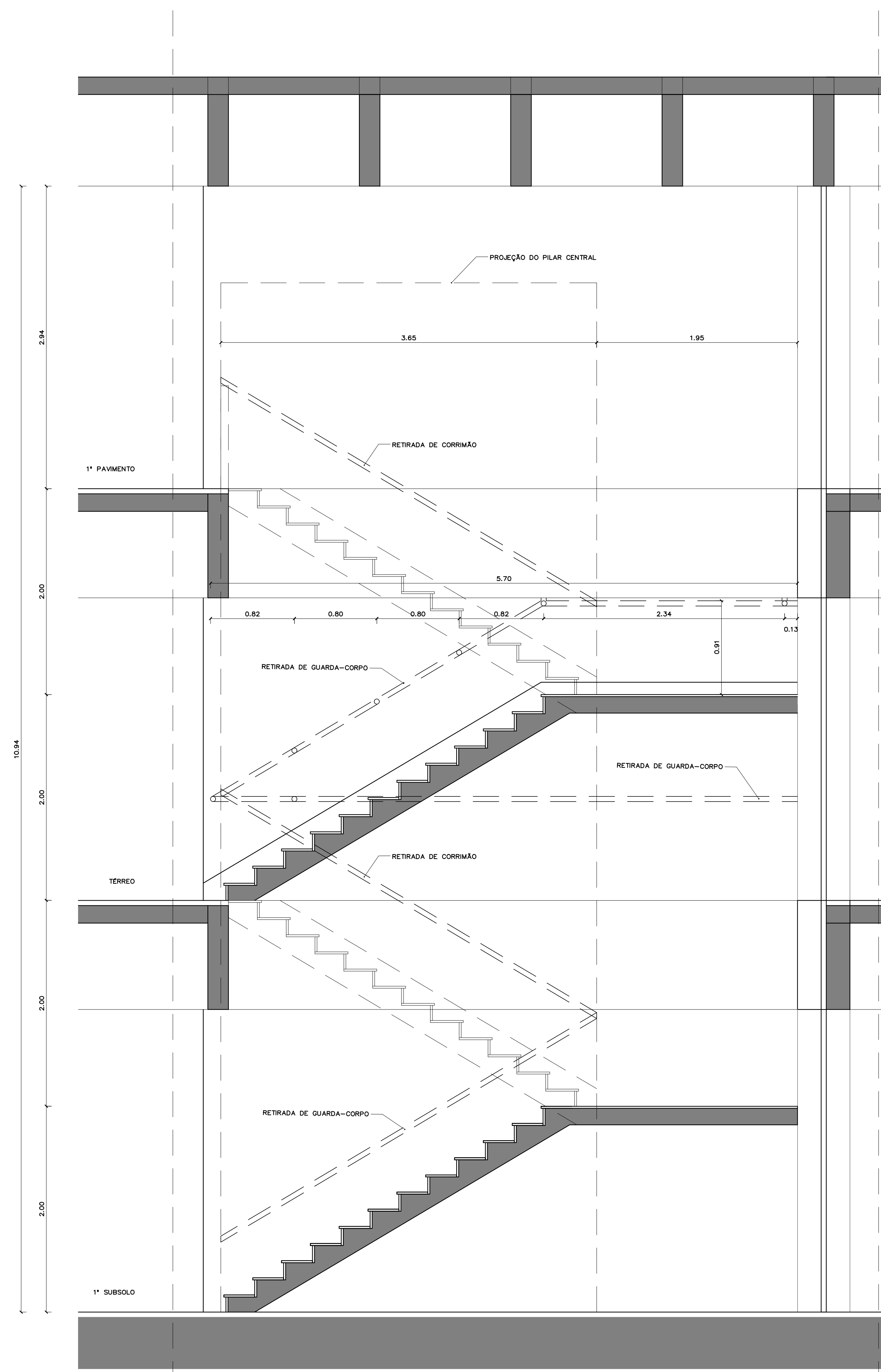
CORTE EE ESCADAS 02 E 03 ESC.: 1:25
