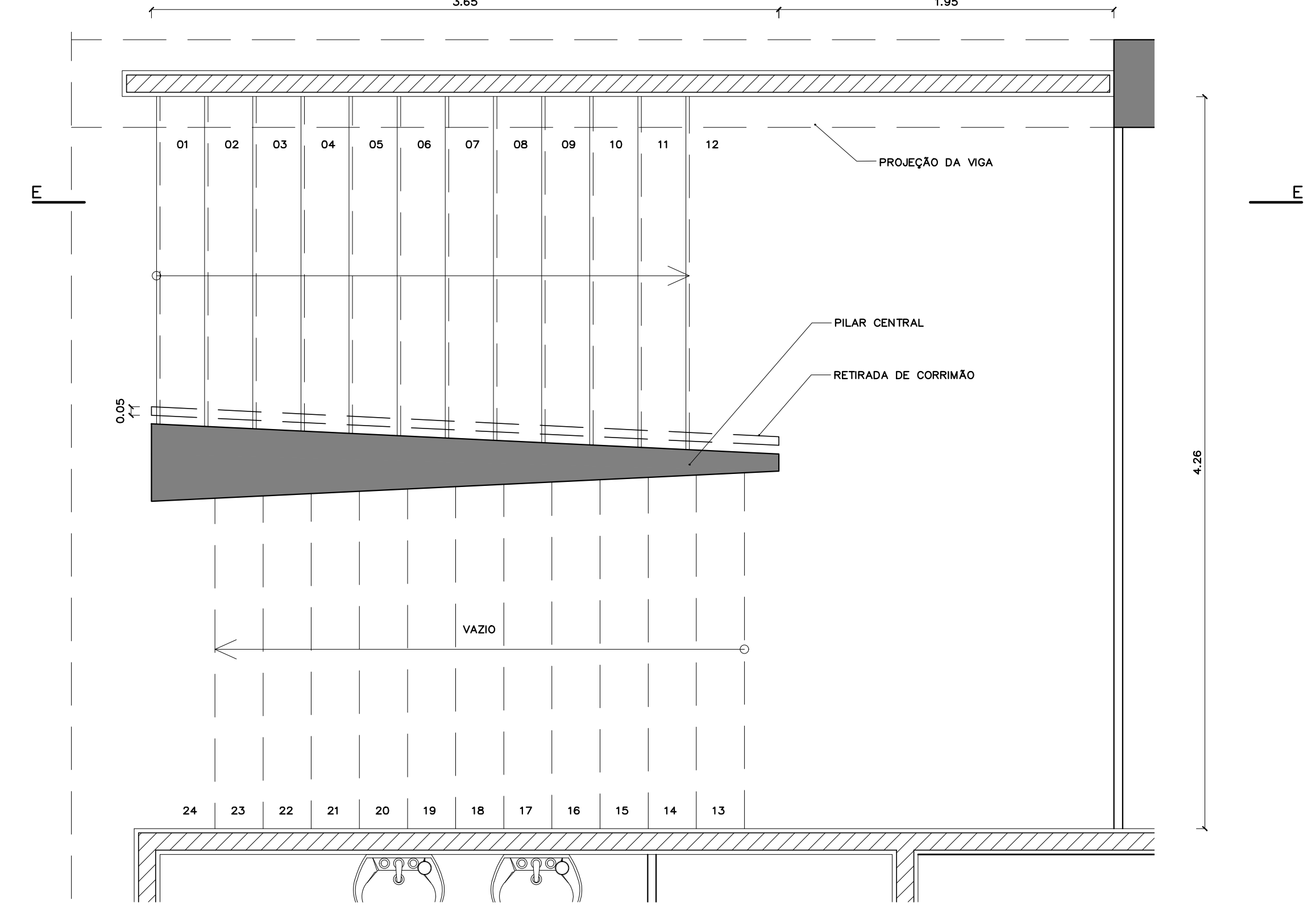
PLANTA DEMOLIR / CONSTRUIR ESCADAS 02 E 03 (1º SUBSOLO) ESC.: 1:25
