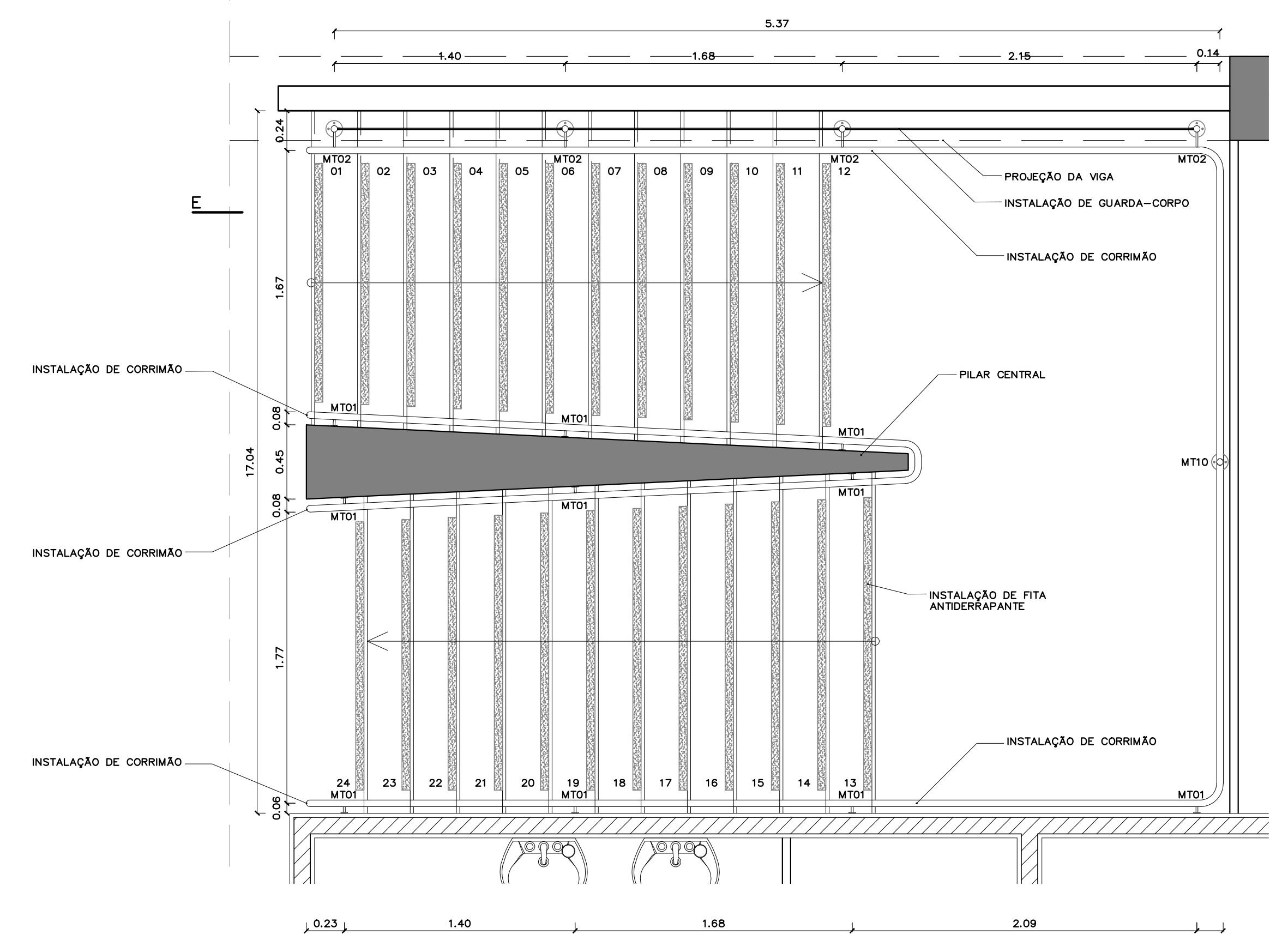
PLANTA BAIXA ESCADAS 02 E 03 (TÉRREO) ESC.: 1:25
