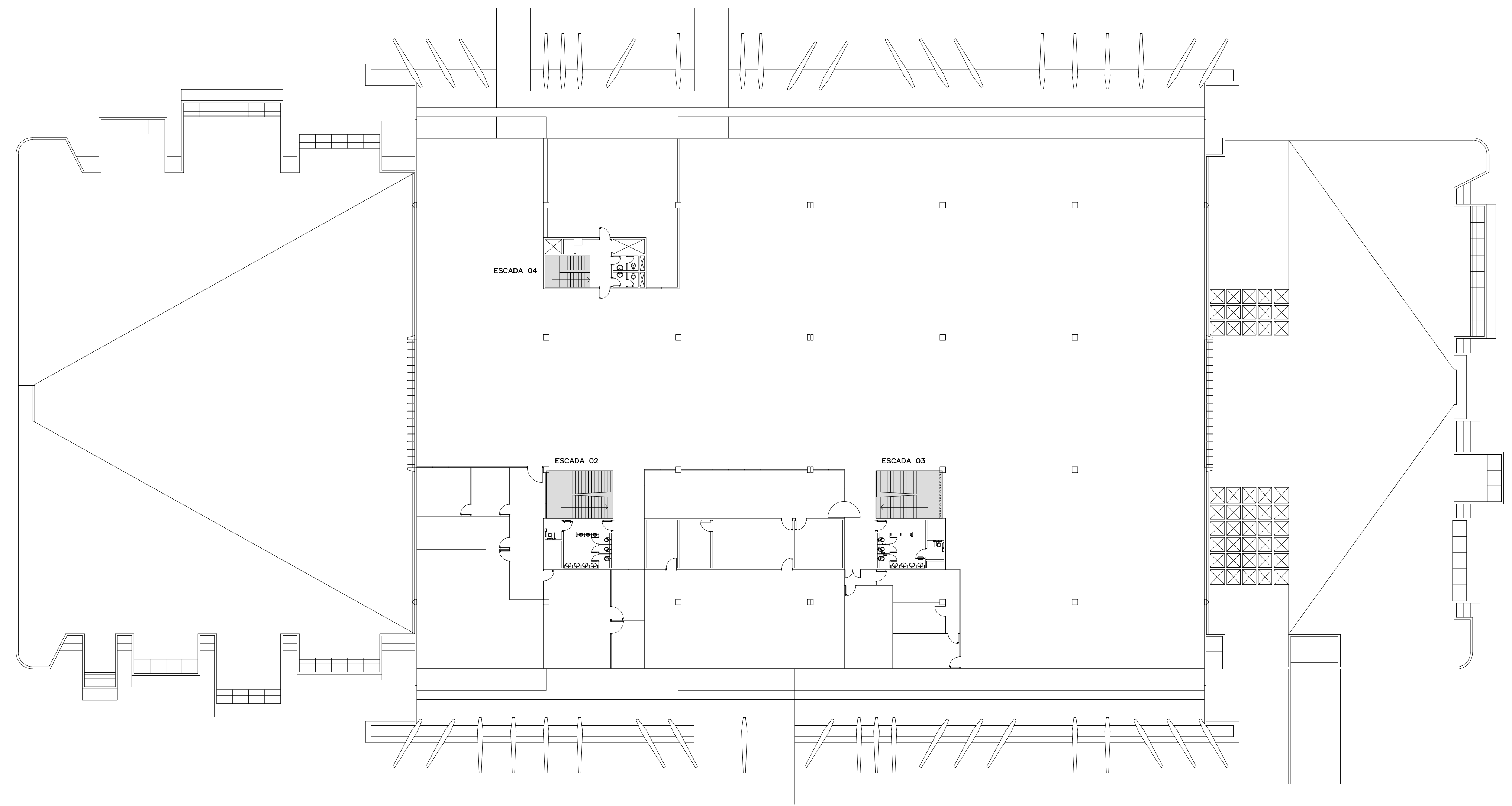
PLANTA DE LOCAÇÃO 1º PAVIMENTO ESC.: 1:250
