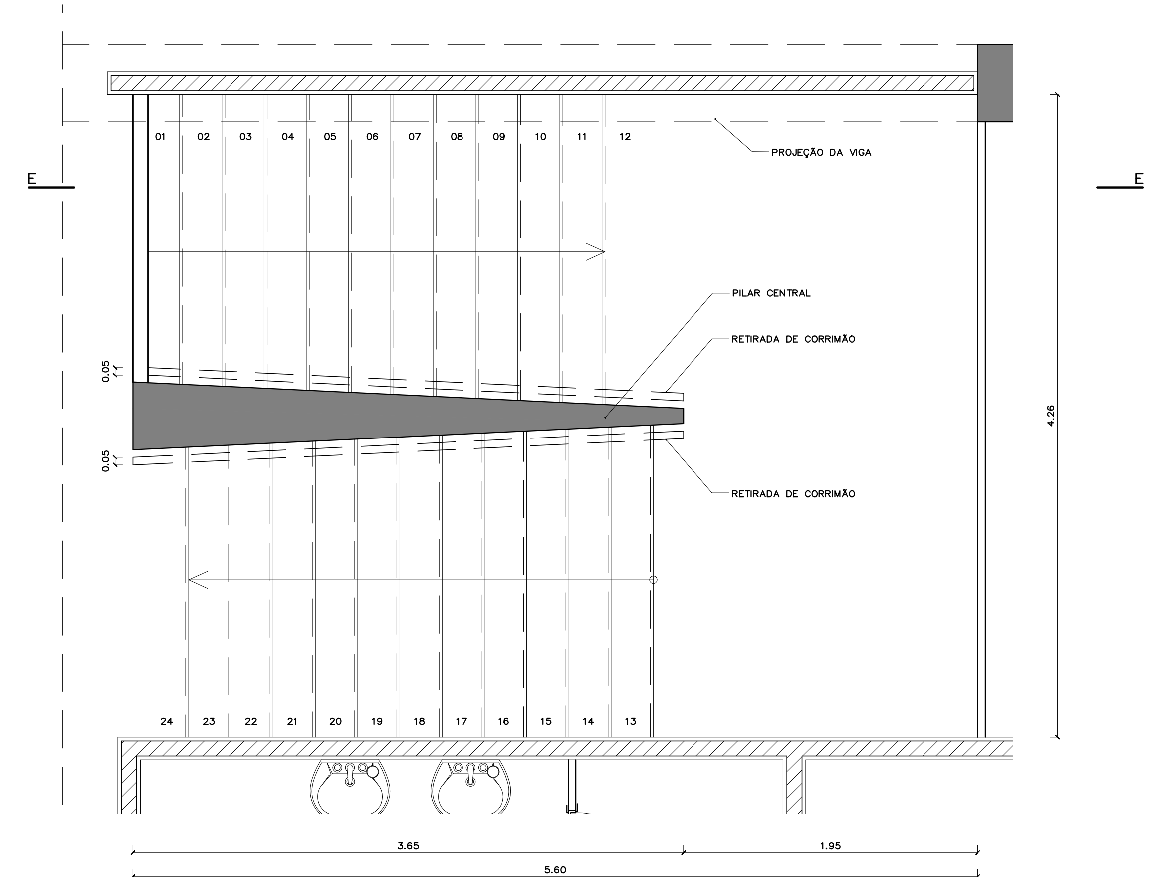
PLANTA DEMOLIR / CONSTRUIR ESCADAS 02 E 03 (1º PAVIMENTO) ESC.: 1:25
