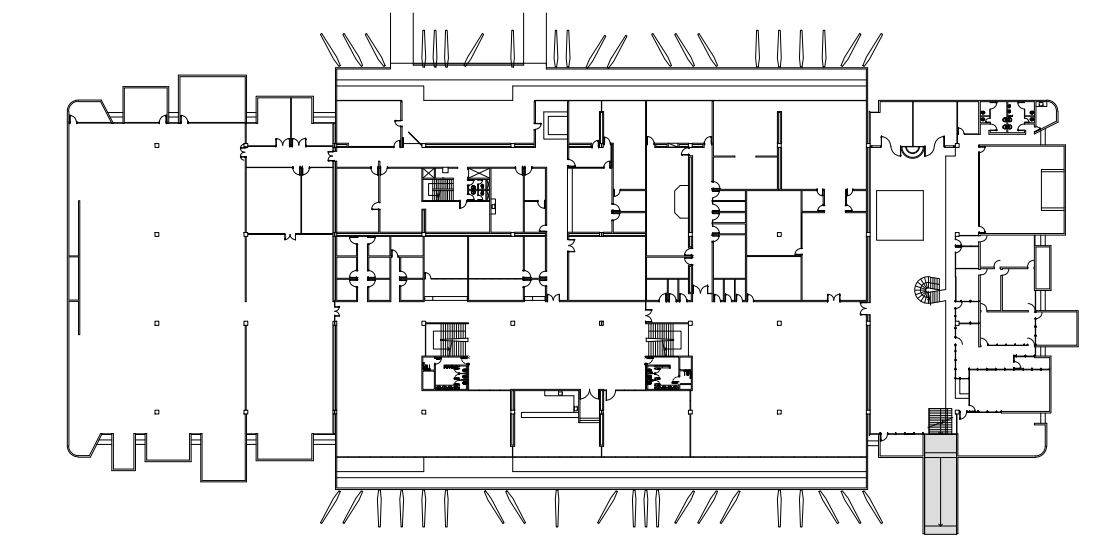
BCE - 1º SUBSOLO ESC: 1:1000
