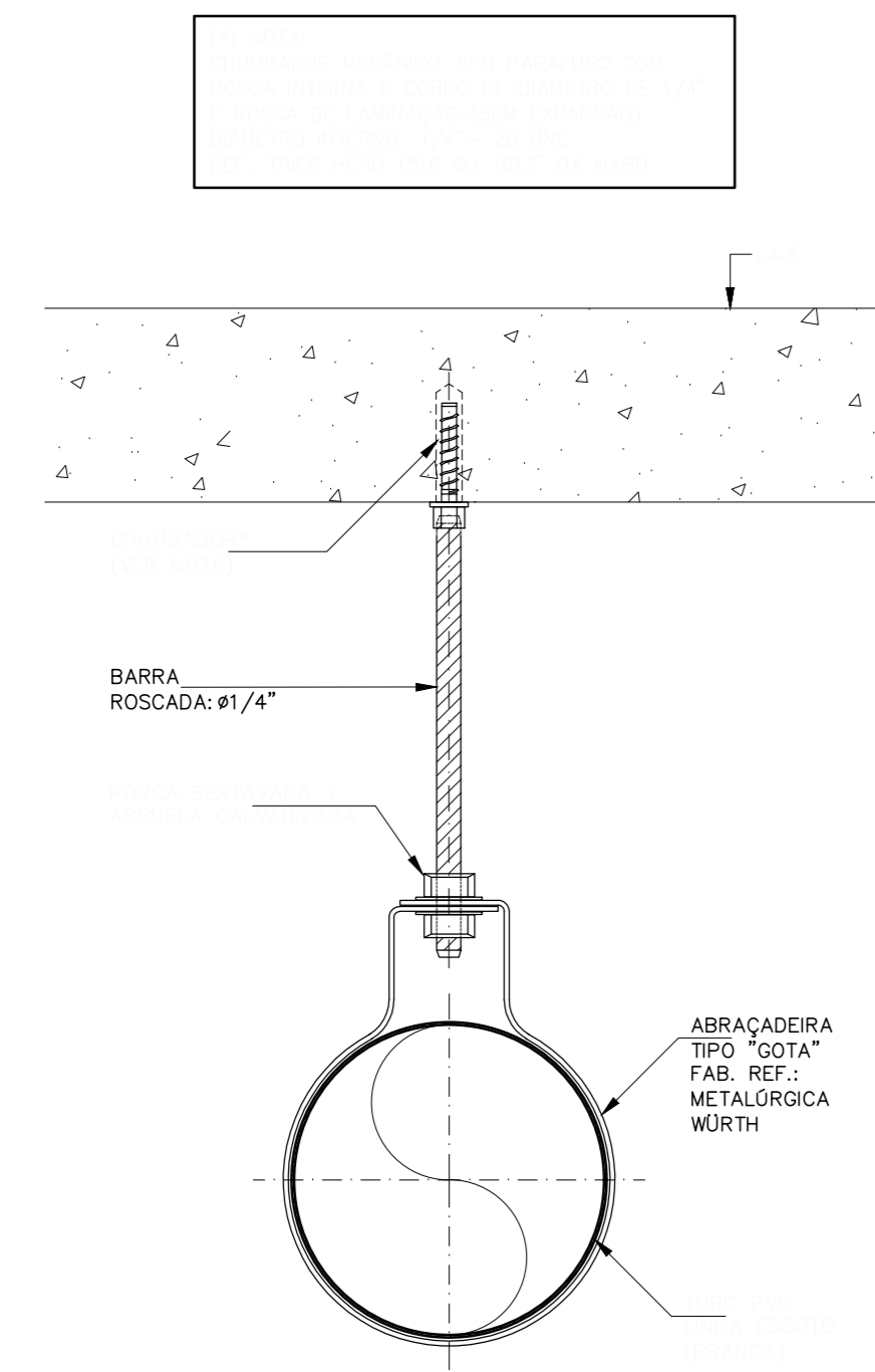
DETALHE TÍPICO DE FIXAÇÃO DE TUBO PVC NA LAJE SEM ESCALA
