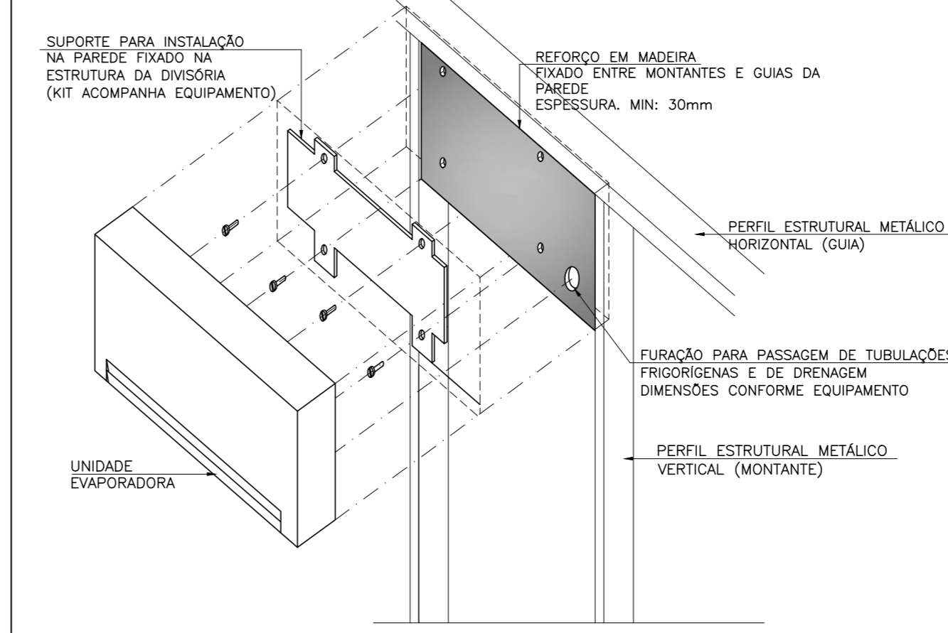
DETALHE DE FIXAÇÃO DA UNIDADE EVAPORADORA COM REFORÇO EM PAREDE TIPO DRY WALL SEM ESCALA
