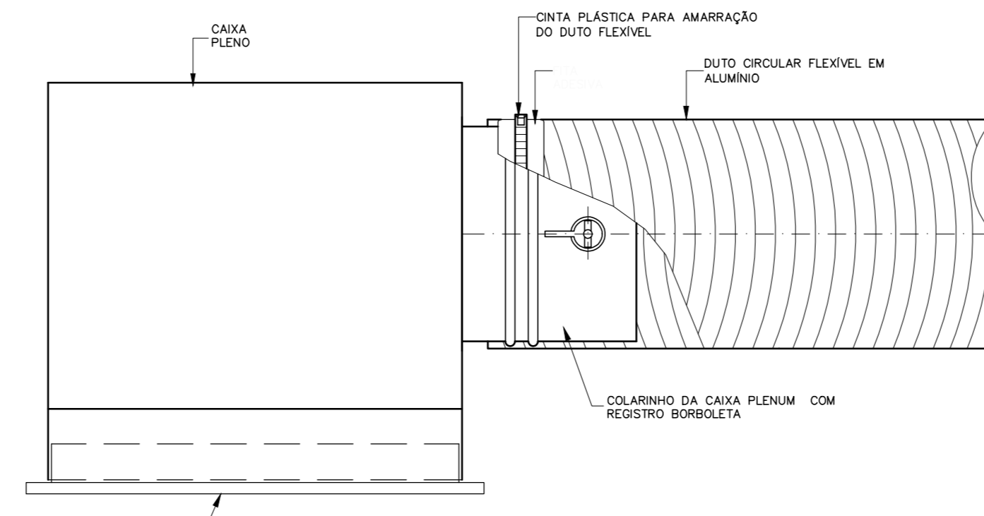
FIXAÇÃO NA GRELHA
