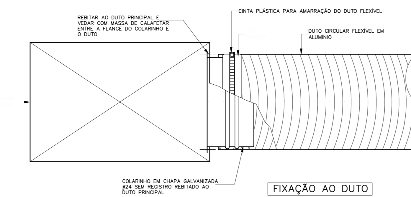
FIXAÇÃO AO DUTO
