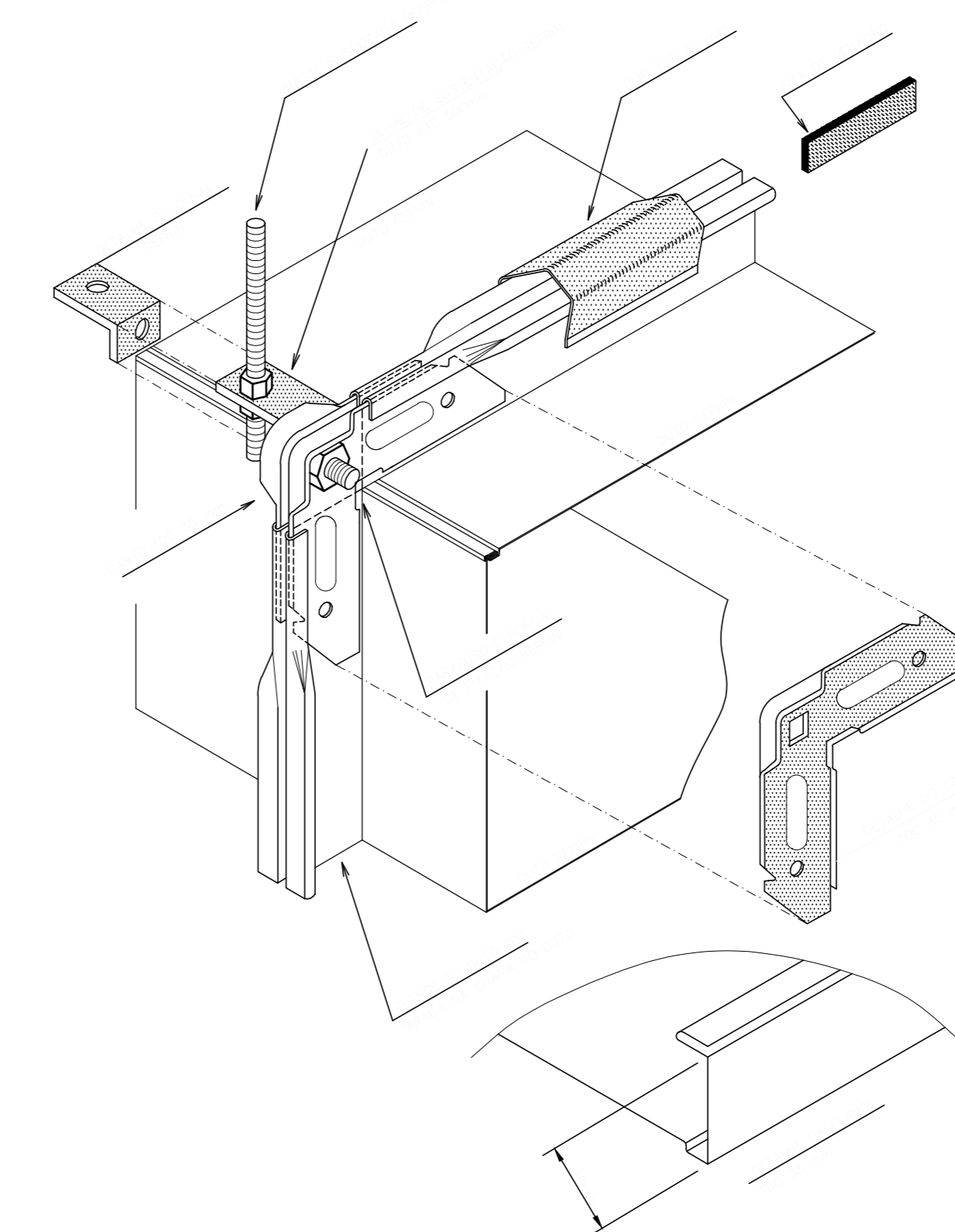
DETALHE DE FLANGES TDC SEM ESCALA / VERSÃO: 1.0
